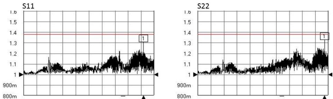
PE3VNA4002-24 VSWR
