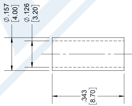
FERRULE
